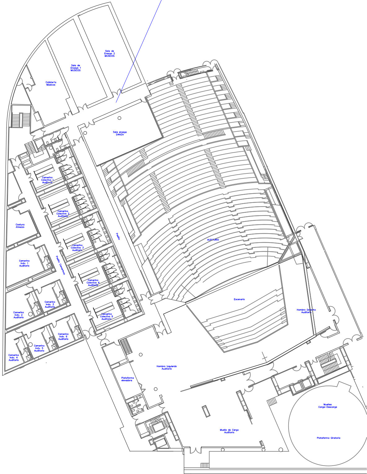
PLANTA SOTANO -1
